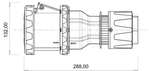
PLANO TÉCNICO
