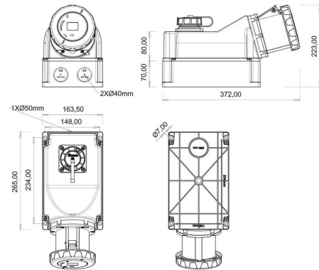
PLANO TÉCNICO
