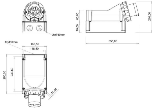
PLANO TÉCNICO
