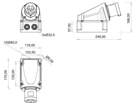
PLANO TÉCNICO
