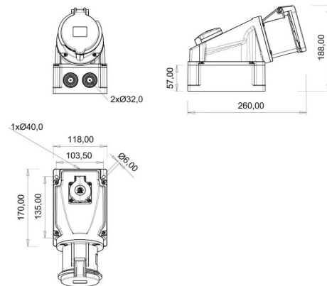
PLANO TÉCNICO
