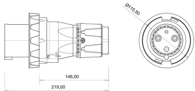
PLANO TÉCNICO
