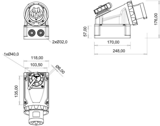
PLANO TÉCNICO
