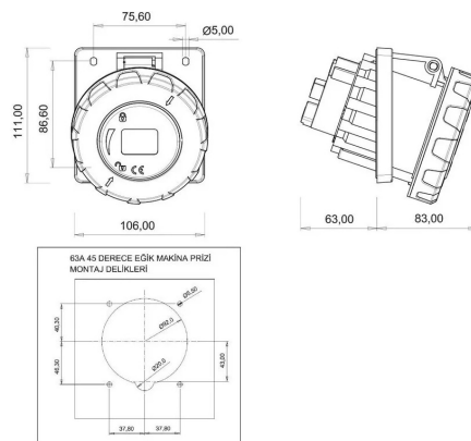
PLANO TÉCNICO
