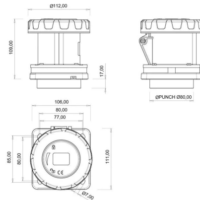
PLANO TÉCNICO
