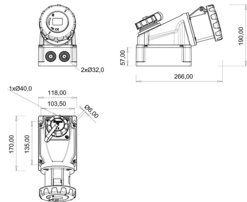
PLANO TÉCNICO
