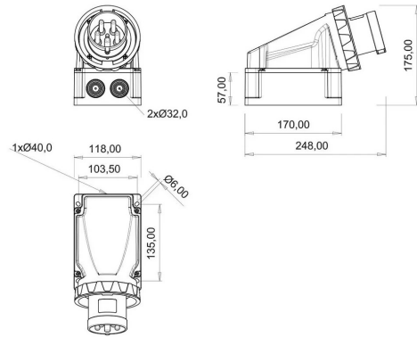
PLANO TÉCNICO
