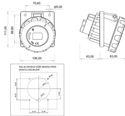
PLANO TÉCNICO
