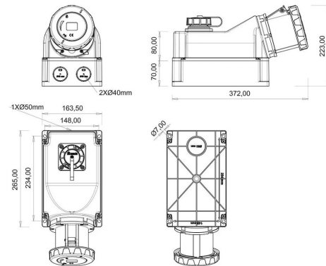
PLANO TÉCNICO
