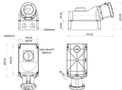
PLANO TÉCNICO
