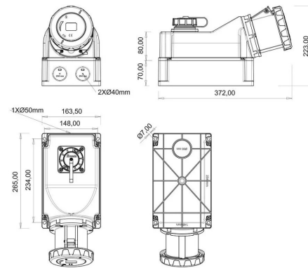
PLANO TÉCNICO
