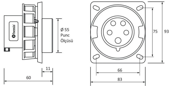
PLANO TÉCNICO
