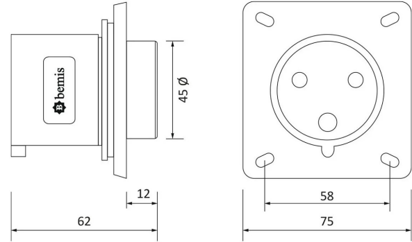
PLANO TÉCNICO
