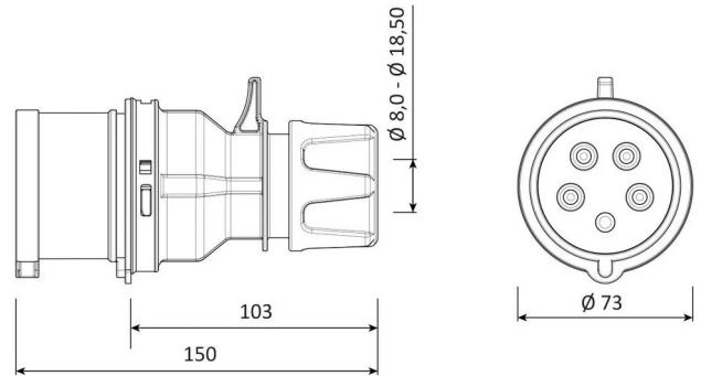
PLANO TÉCNICO
