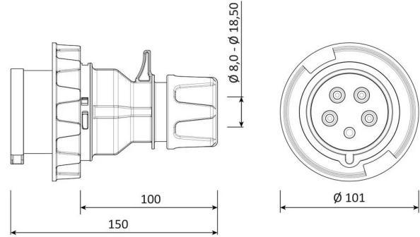
PLANO TÉCNICO
