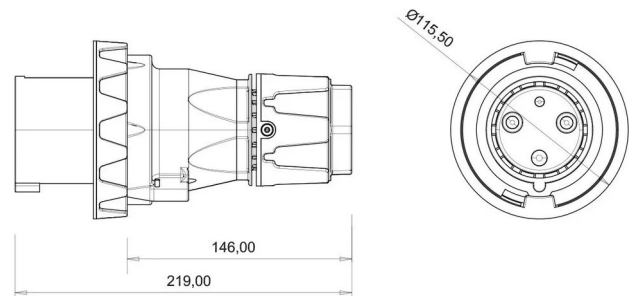
PLANO TÉCNICO
