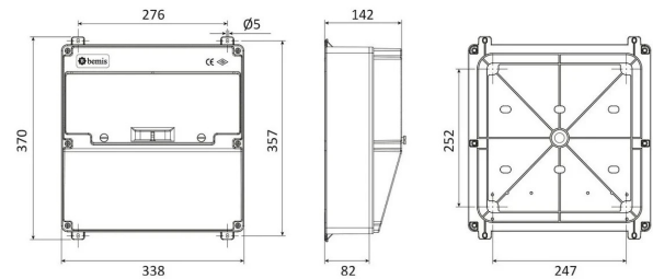
PLANO TÉCNICO
