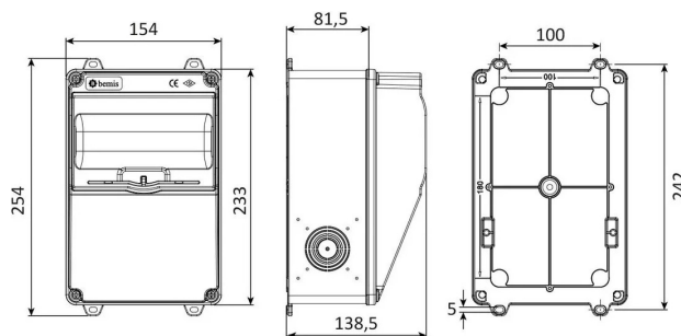
PLANO TÉCNICO
