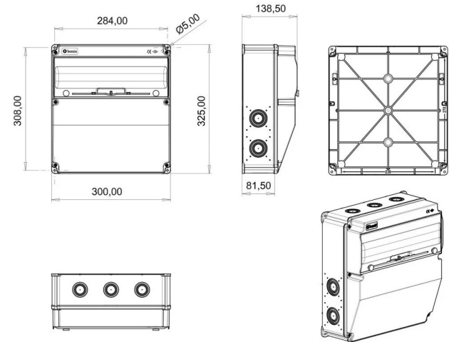
PLANO TÉCNICO
