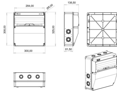
PLANO TÉCNICO
