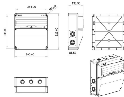
PLANO TÉCNICO
