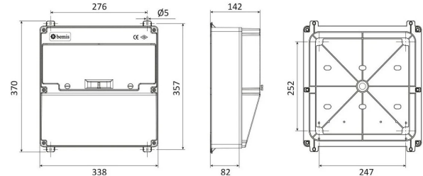
PLANO TÉCNICO
