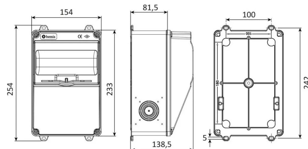
PLANO TÉCNICO
