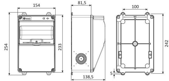
PLANO TÉCNICO
