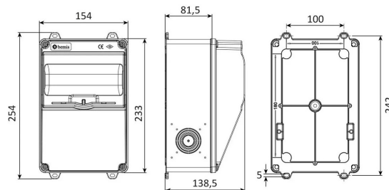
PLANO TÉCNICO
