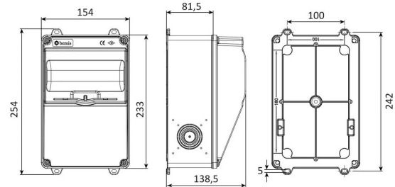
PLANO TÉCNICO
