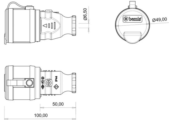
PLANO TÉCNICO
