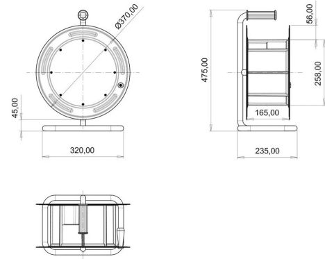
PLANO TÉCNICO
