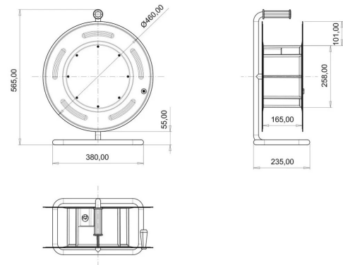
PLANO TÉCNICO
