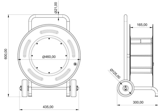
PLANO TÉCNICO
