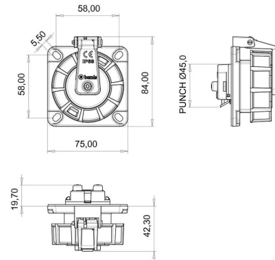
PLANO TÉCNICO
