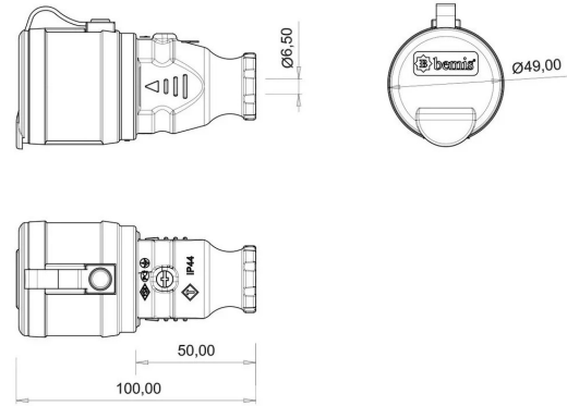
PLANO TÉCNICO
