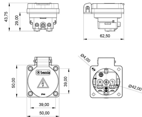
PLANO TÉCNICO
