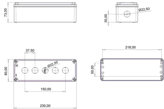
PLANO TÉCNICO
