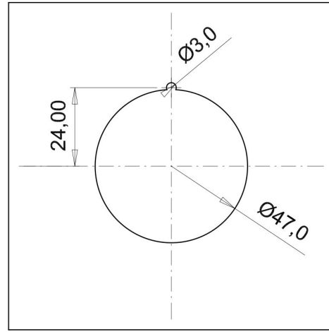
SOMUNLU PANO PRİZİ MONTAJ DELİĞİ ÖLÇÜLERİ
