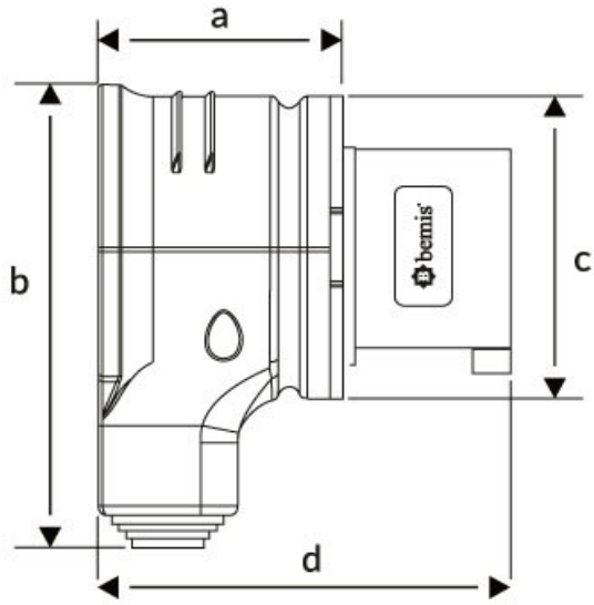
Ölçüler / Dimensions (mm)
