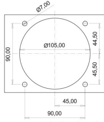
PUNCH DELİK ÖLÇÜLERİ
