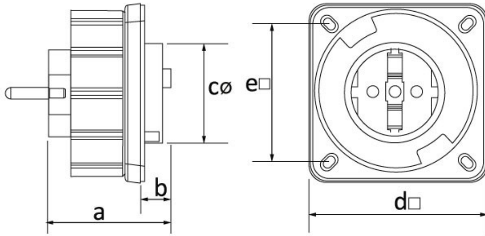
Ölçüler / Dimensions (mm)
