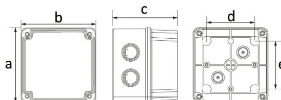
ГАБАРИТНЫЙ ЧЕРТЁЖ
