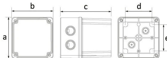
ГАБАРИТНЫЙ ЧЕРТЁЖ
