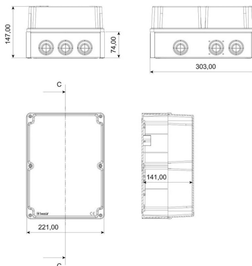
ГАБАРИТНЫЙ ЧЕРТЁЖ
