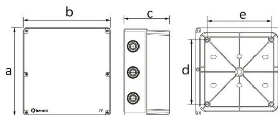
ГАБАРИТНЫЙ ЧЕРТЁЖ
