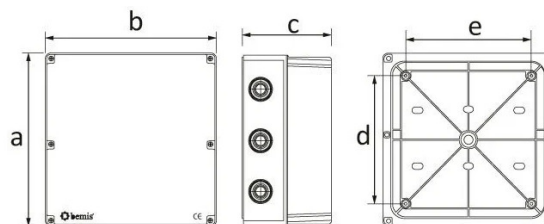
ГАБАРИТНЫЙ ЧЕРТЁЖ
