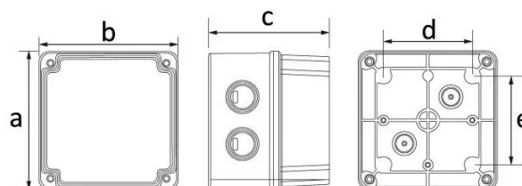
ГАБАРИТНЫЙ ЧЕРТЁЖ
