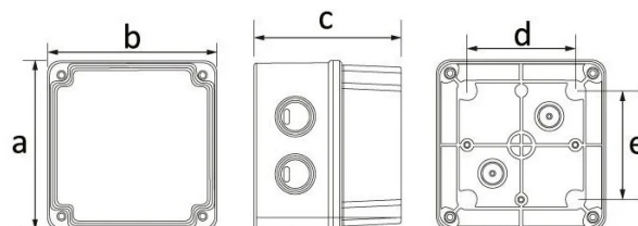
ГАБАРИТНЫЙ ЧЕРТЁЖ
