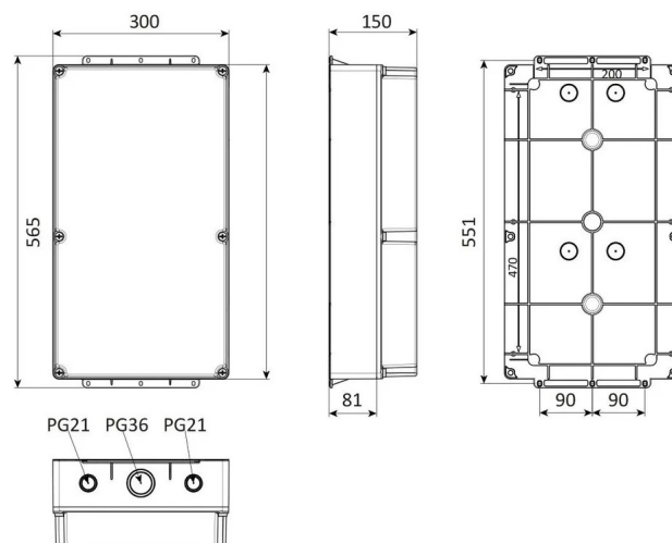
ГАБАРИТНЫЙ ЧЕРТЁЖ
